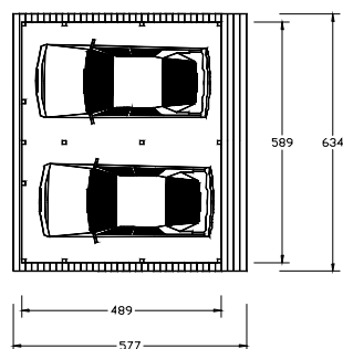
Draufsicht Art.-Nr. 4208
