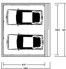
Draufsicht Art.-Nr. 4210
